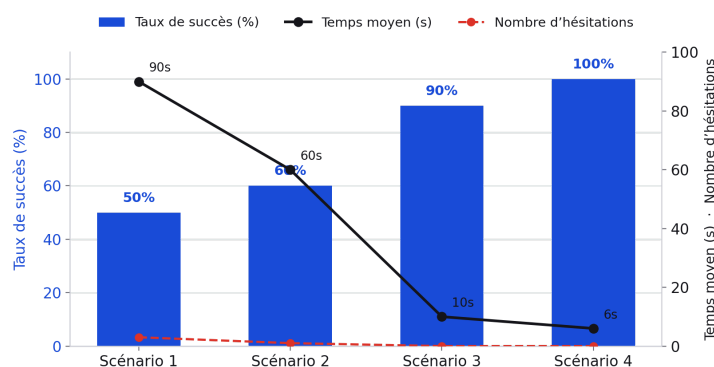
[FIG] Taux de succès (barres), temps moyen et nombre d'hésitations (courbes) par scénario.
