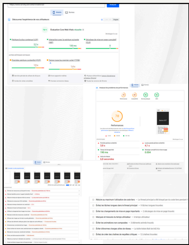
[FIG] Rapports complets PageSpeed Insights de la page « Notre IUT ».
